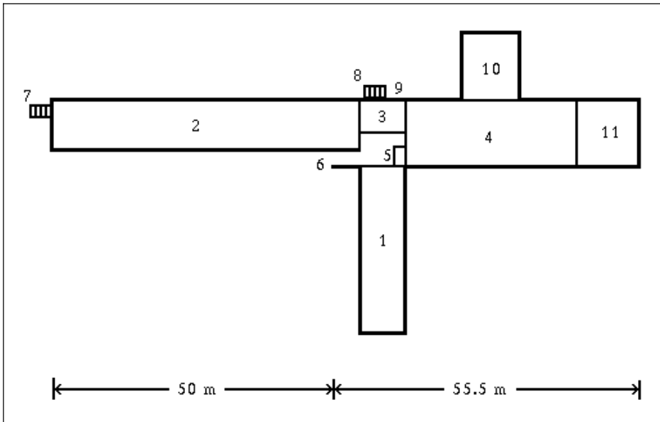
Fig. 33: Plan of Auschwitz Crematorium II.
