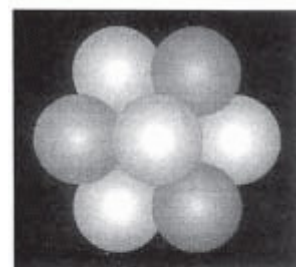
Fig. 6-8. Esferas tridimensionales
