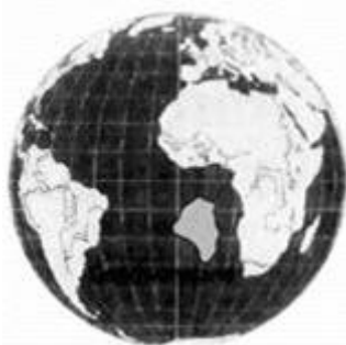
Fig. 3-11. Gondwanalandia
