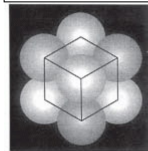
Fig. 6-8a. Conectando los centros para formar un cubo.
