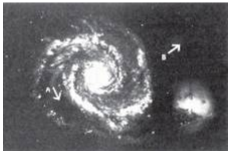
Fig. 2-35. Galaxia espiral
