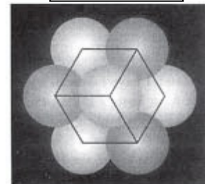
Fig. 6-8a. Conectando los centros para formar un cubo.
