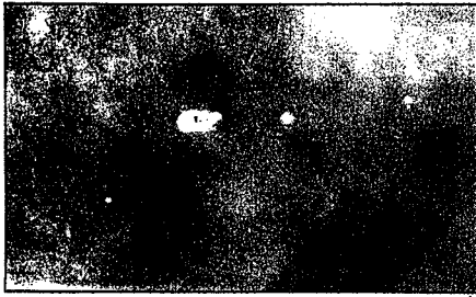
Cinco estrellas jóvenes en la nebulosa de Orión, vistas con el Hubble . Alrededor de cuatro de ellas, posibles discos protoplanetarios.
